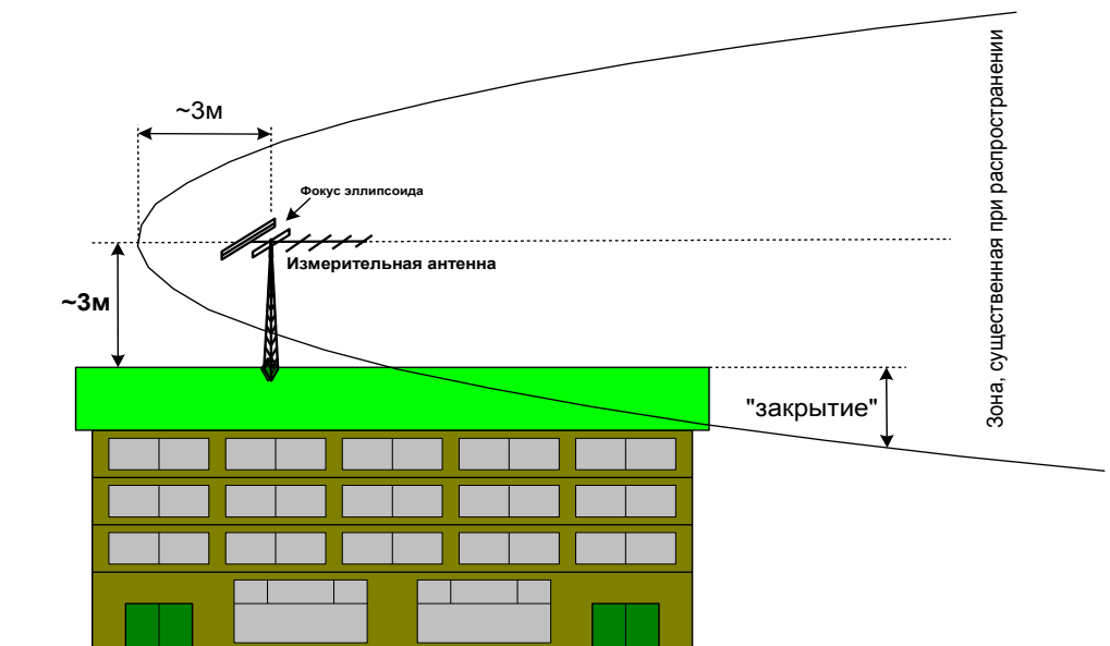
Рисунок Е.11 – Зона, существенная при распространении.
