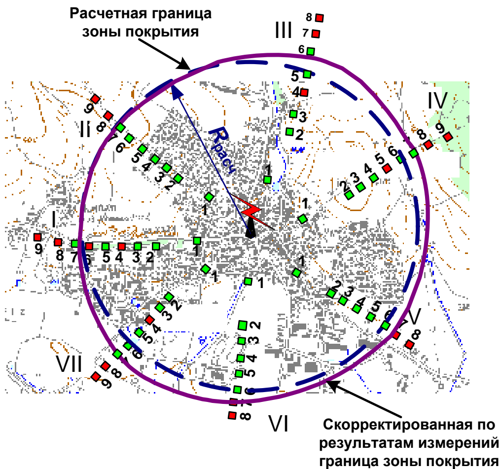
Рисунок 6 – Пример представления скорректированной границы зоны покрытия.
