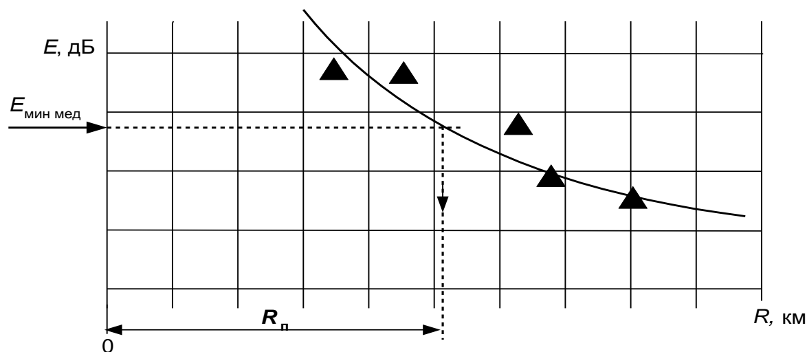
Рисунок Е.7 – Медианные значения напряженности поля в малых зонах (треугольники) и использование экспериментальной кривой для нахождения радиуса зоны покрытия по данным измерений.
