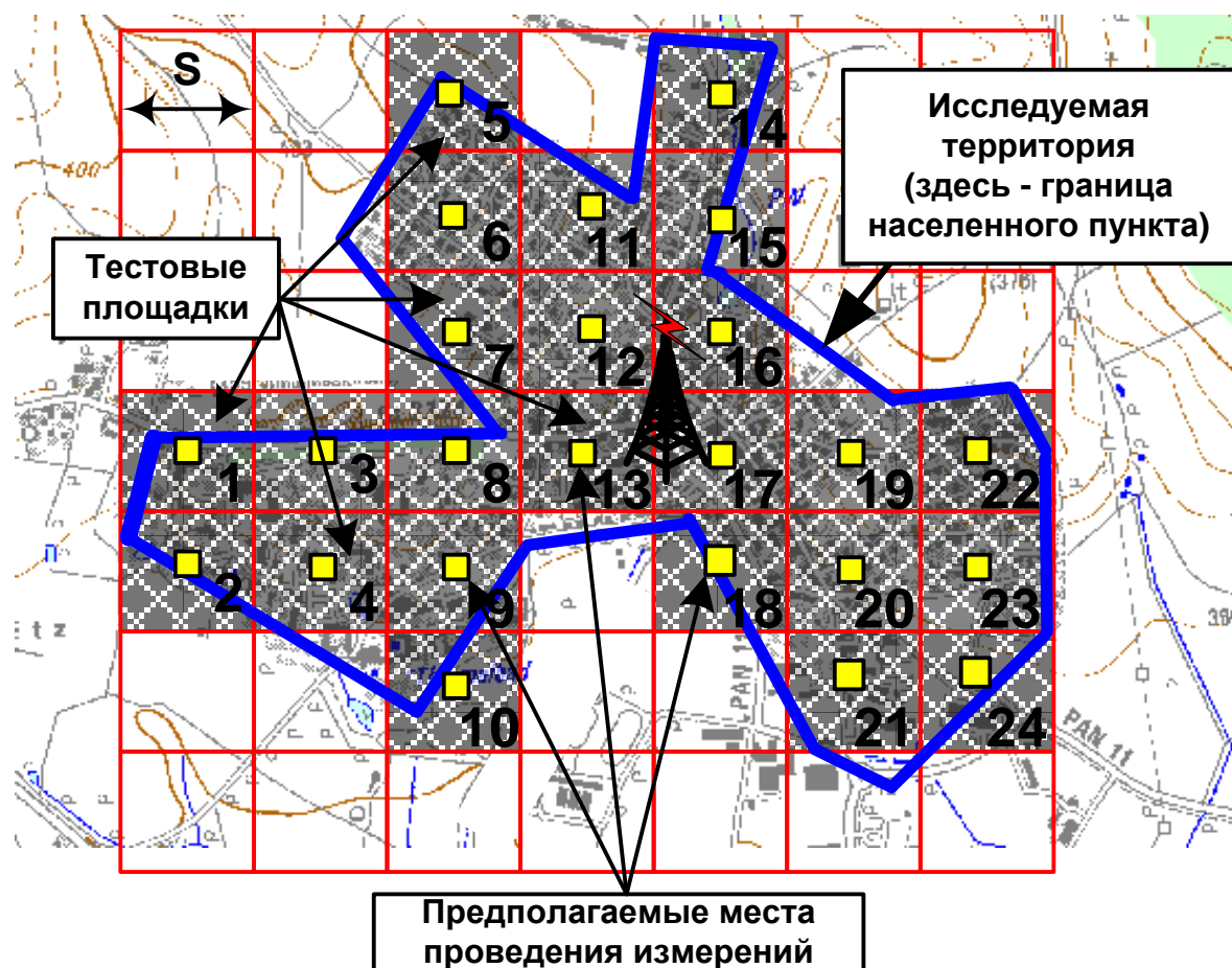
Рисунок 7 – Пример размещения сетки и плановых мест приема внутри исследуемой зоны.
