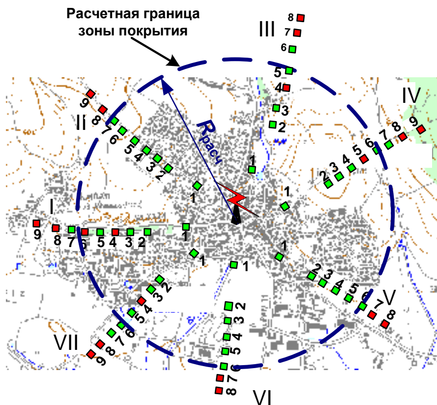
Рисунок 4 – Пример представления обработанных результатов измерений по направлениям.
