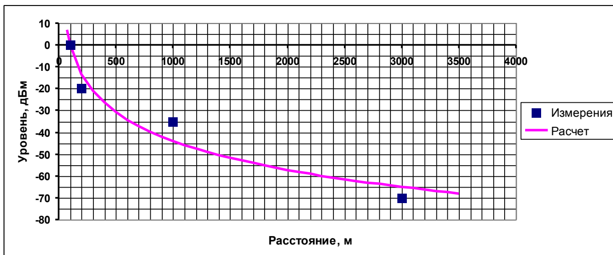
Рисунок Е.8 – Пример графического представления кривой P(d_2) .
