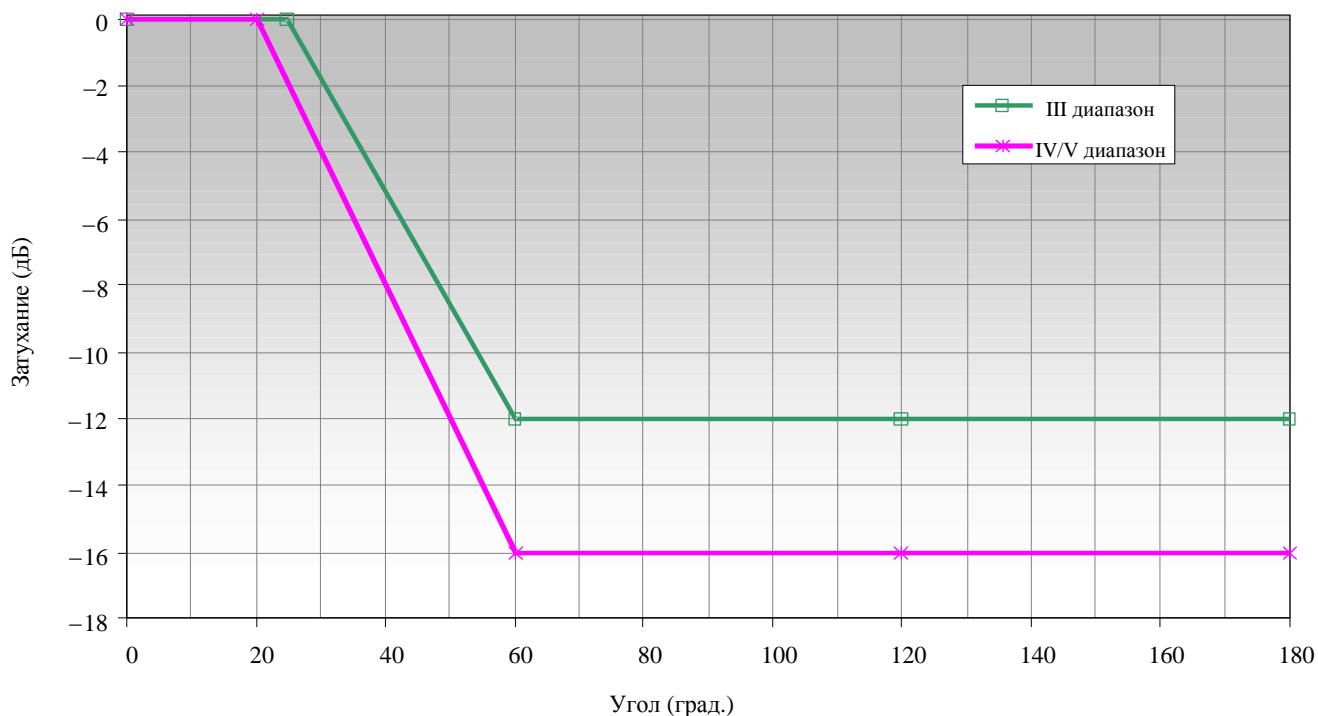
Рисунок 1 – Диаграмма направленности приемной направленной антенны.
