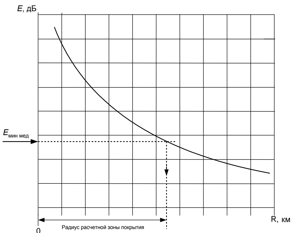
Рисунок Е.5 – Нахождение радиуса зоны покрытия по расчетной кривой E(R) вдоль одного из направлений при удалении от передатчика.
