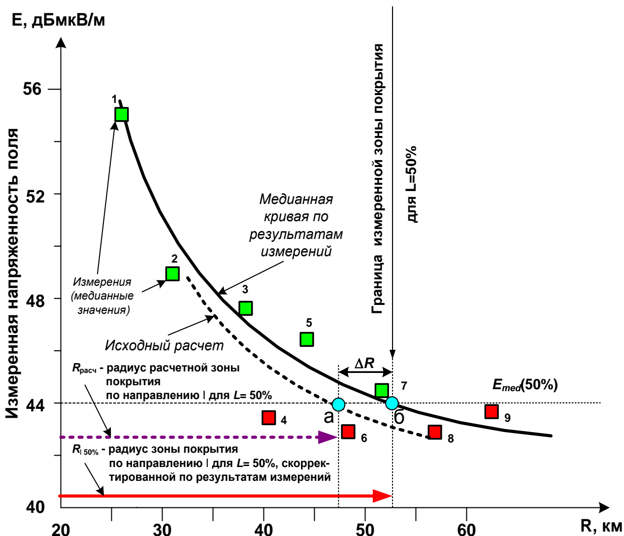
Рисунок 5 – Пример обработки результатов измерений на одном из направлений при определении границы зоны покрытия для вероятности охвата 50% мест.
