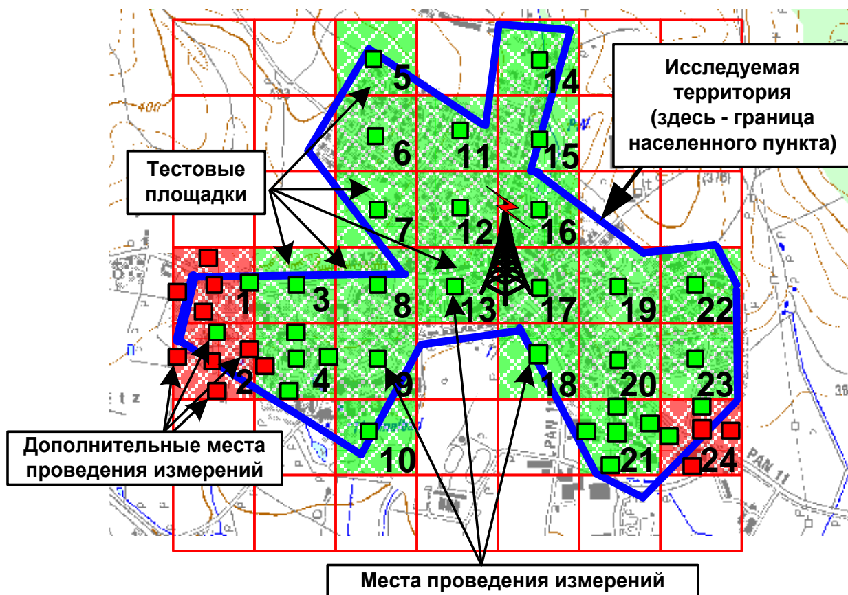
Рисунок 8 – Пример представления результатов измерений.
