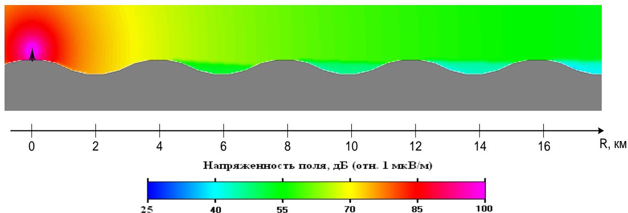
Рисунок Е.16 – Распределение напряженности поля сигнала по заданному направлению
