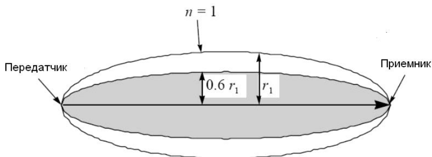
Рисунок Е.12 – Область существенная для распространения радиоволны.
