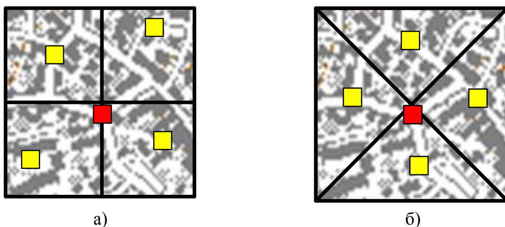
Рисунок Е.20 – Пример выбора в населенном пункте 4 дополнительных мест приема внутри одной тестовой площадки.
